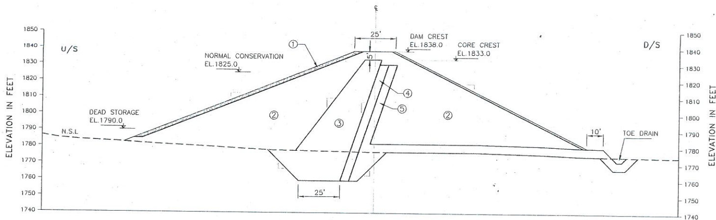
SECTION D-D
