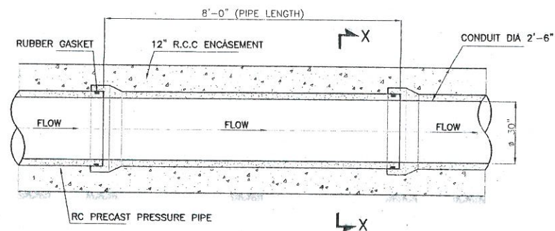
IRRIGATION CONDUIT DETAIL (TYP.)
