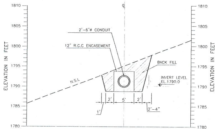
SECTION D-D
