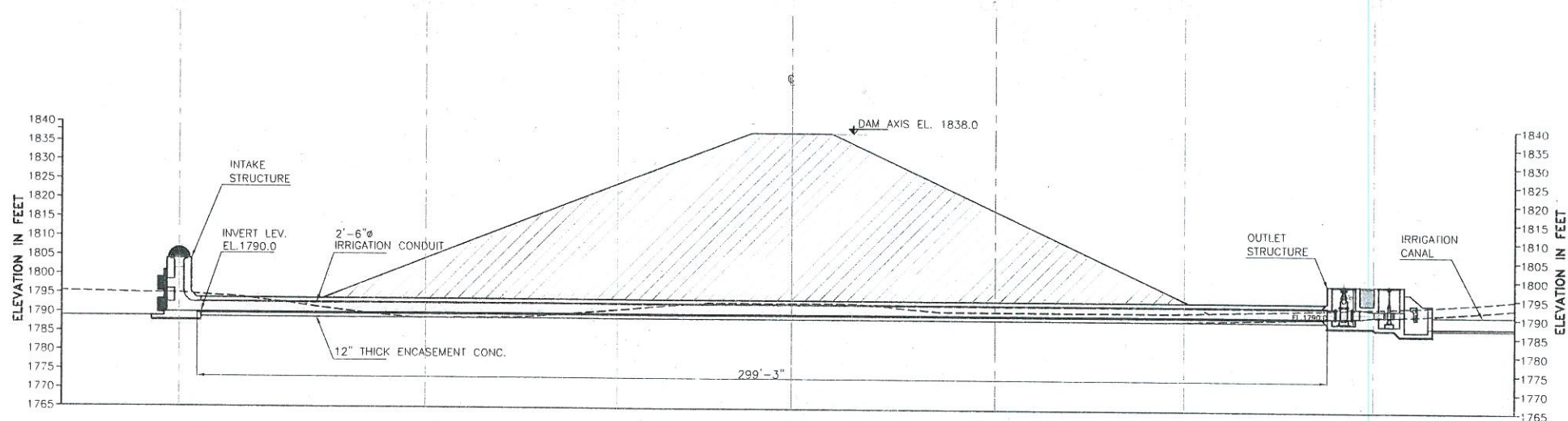
LONGITUDINAL SECTION A-A
