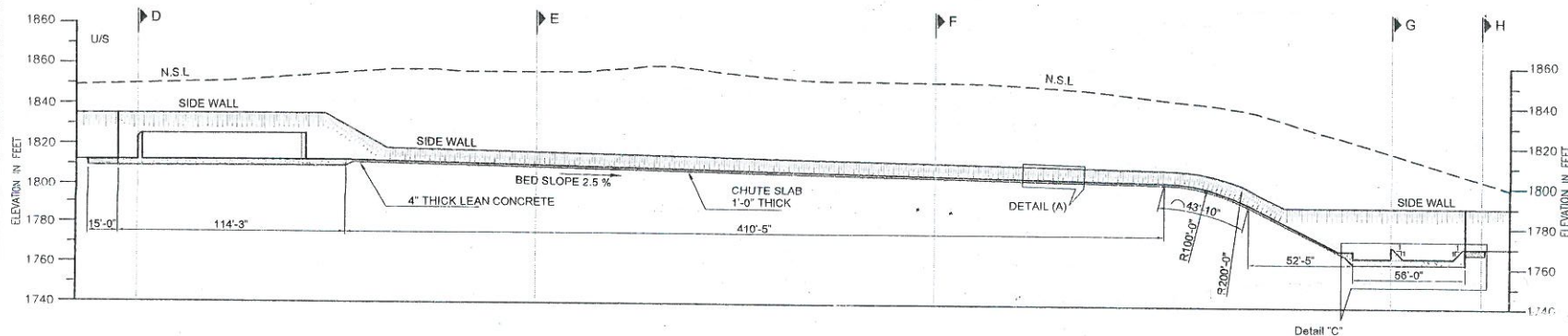
SECTION A-A
